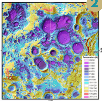
Gemiddelde oppervlaktetemperaturen op de zuidpool van de maan waar de trillings-sensoren in de permanente schaduwen van 40 K laten zien.
