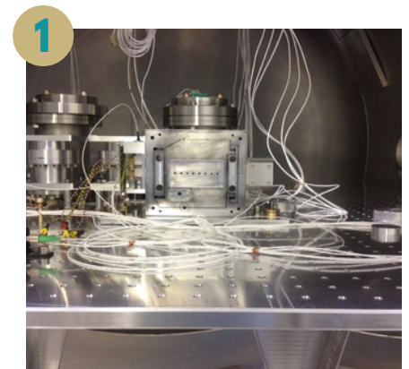
1 Een trillingssensor met precisie laserinterferometer uitlezing. In het frame is een massa opgehangen en deze volgt het frame niet. De uitlezing zit vast aan het frame en meet de beweging van de massa en dus de trillingen van het oppervlak waarop het frame staat, in dit geval de optische tafel.
